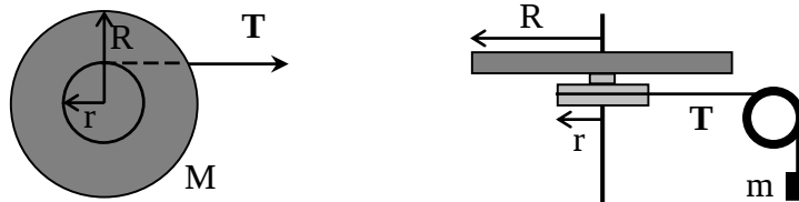
Figura 1. Izquierda: vista superior del disco rotatorio. Derecha: vista lateral, con el sistema de poleas y masa colgante.
