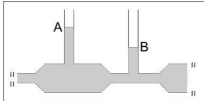
Figura 2: dispositivo utilizado
