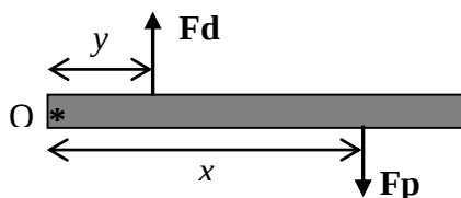
Figura 2. Esquema de la barra pivotada en O.
